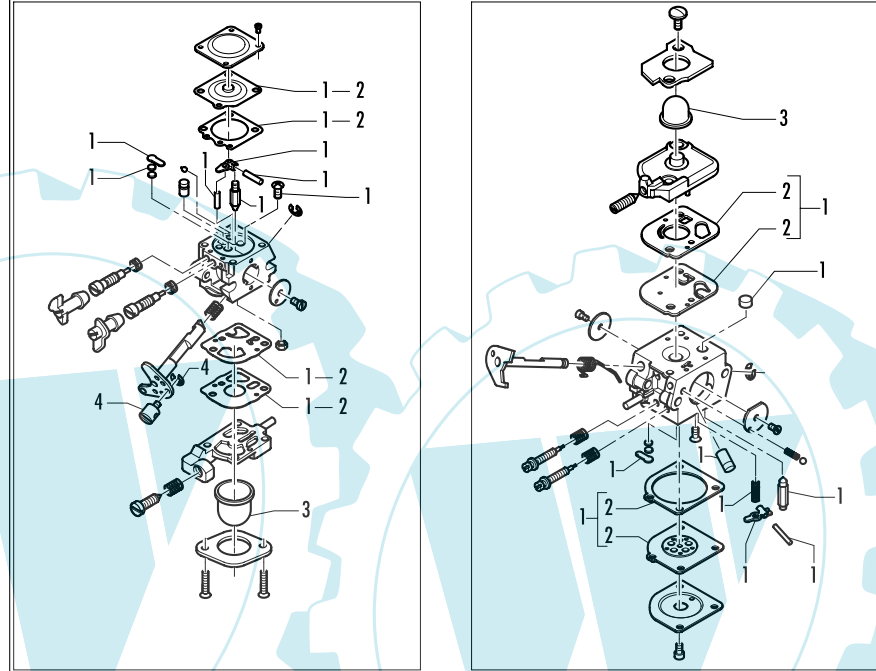
WALBRO WT 547
